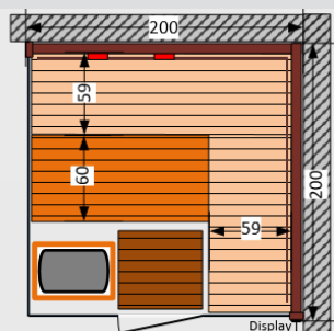
Design: KITZBÜHEL 200 Standard rechts Außenmaße: 200 x 200 x 200 cm (inkl. ca. 3 cm Hinterlüftung); IR-Rotlicht- oder Keramikstrahler sind optional
