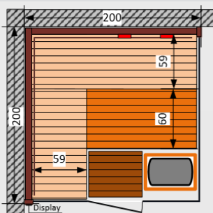
Design: KITZBÜHEL 200 Standard links Außenmaße: 200 x 200 x 200 cm (inkl. ca. 3 cm Hinterlüftung); IR-Rotlicht- oder Keramikstrahler sind optional!
